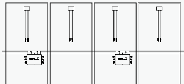
Installationsort des Mikro-Wechselrichters (Rückseite des Solarmoduls)
